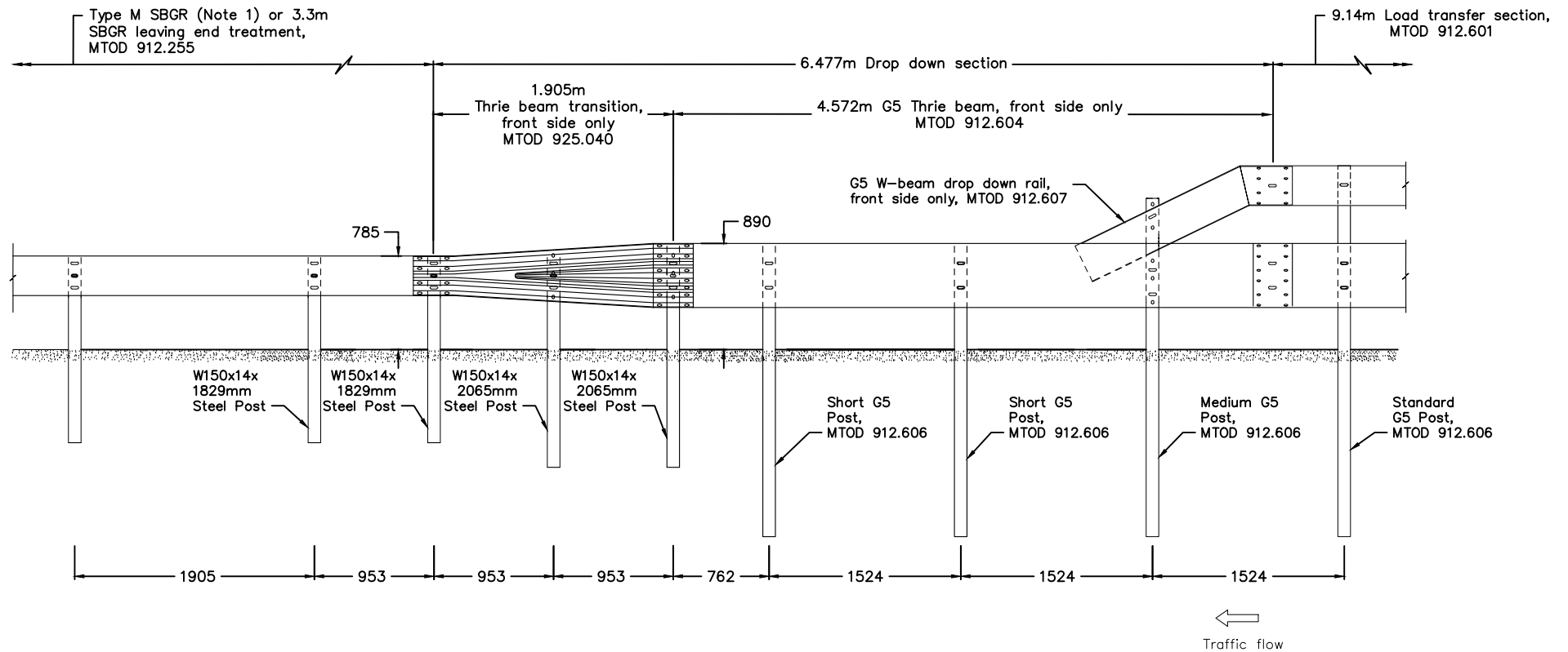
ELEVATION
